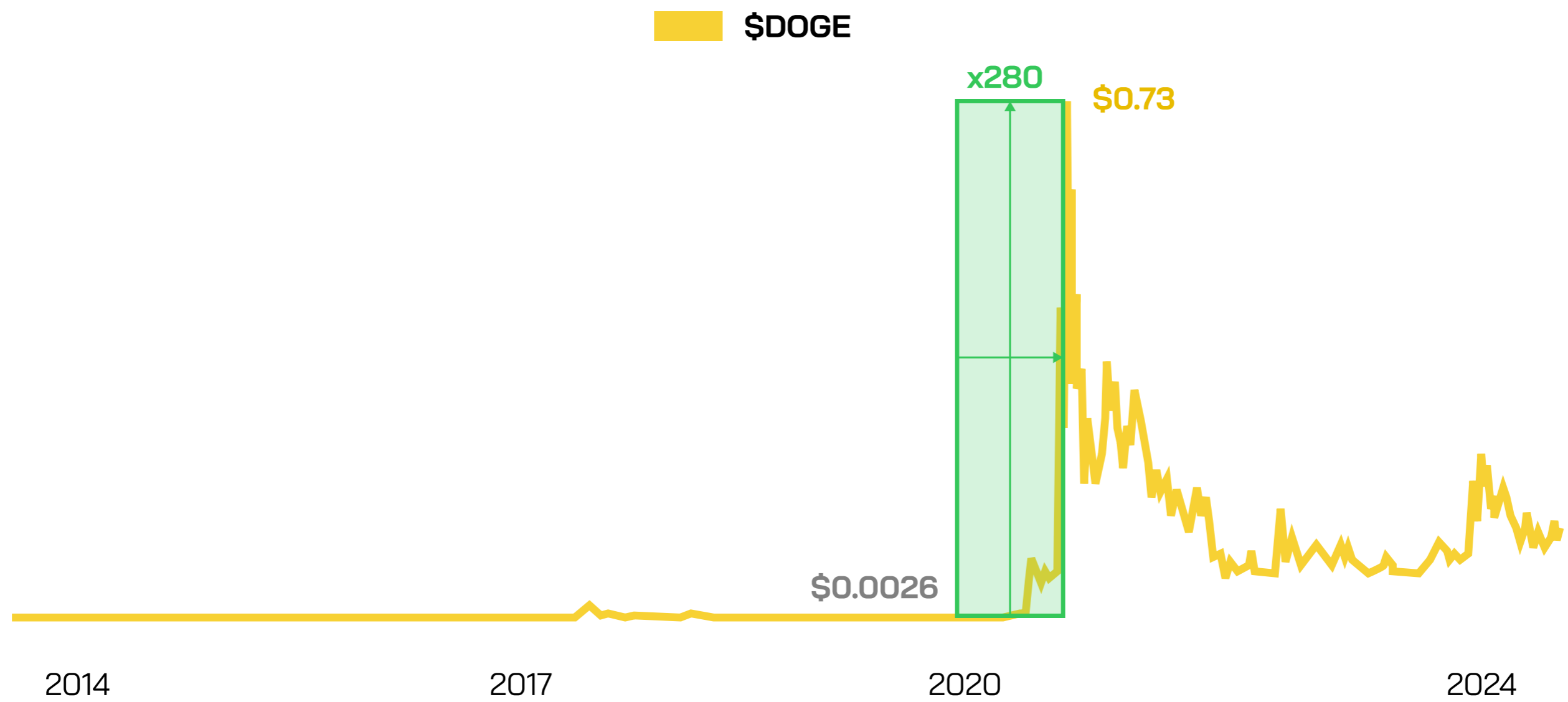
Hình 2: Hiệu suất của $DOGE từ năm 2020 đến 2021
