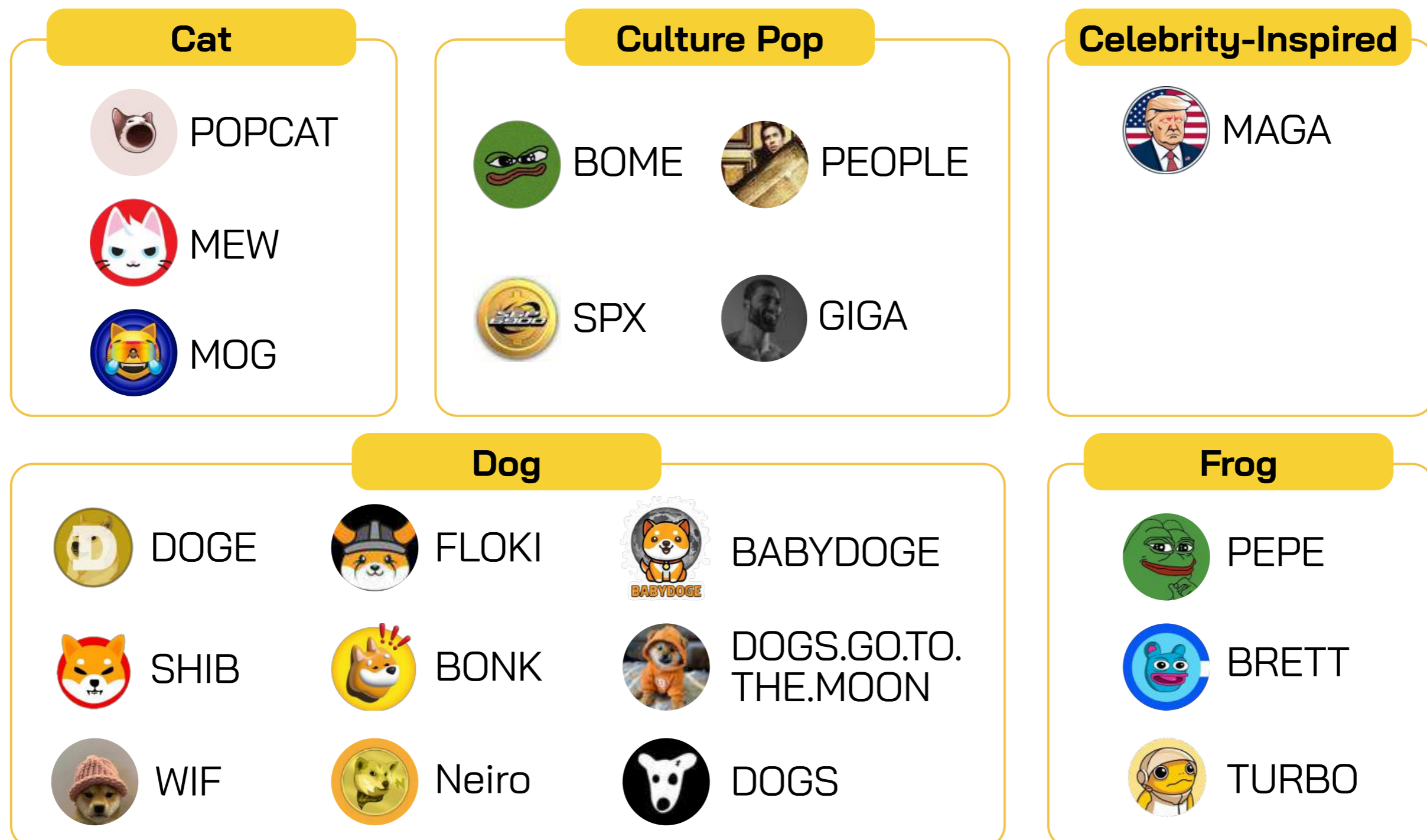
Hình 12: Meme coin có vốn hoá lớn nhất theo chủ đề
