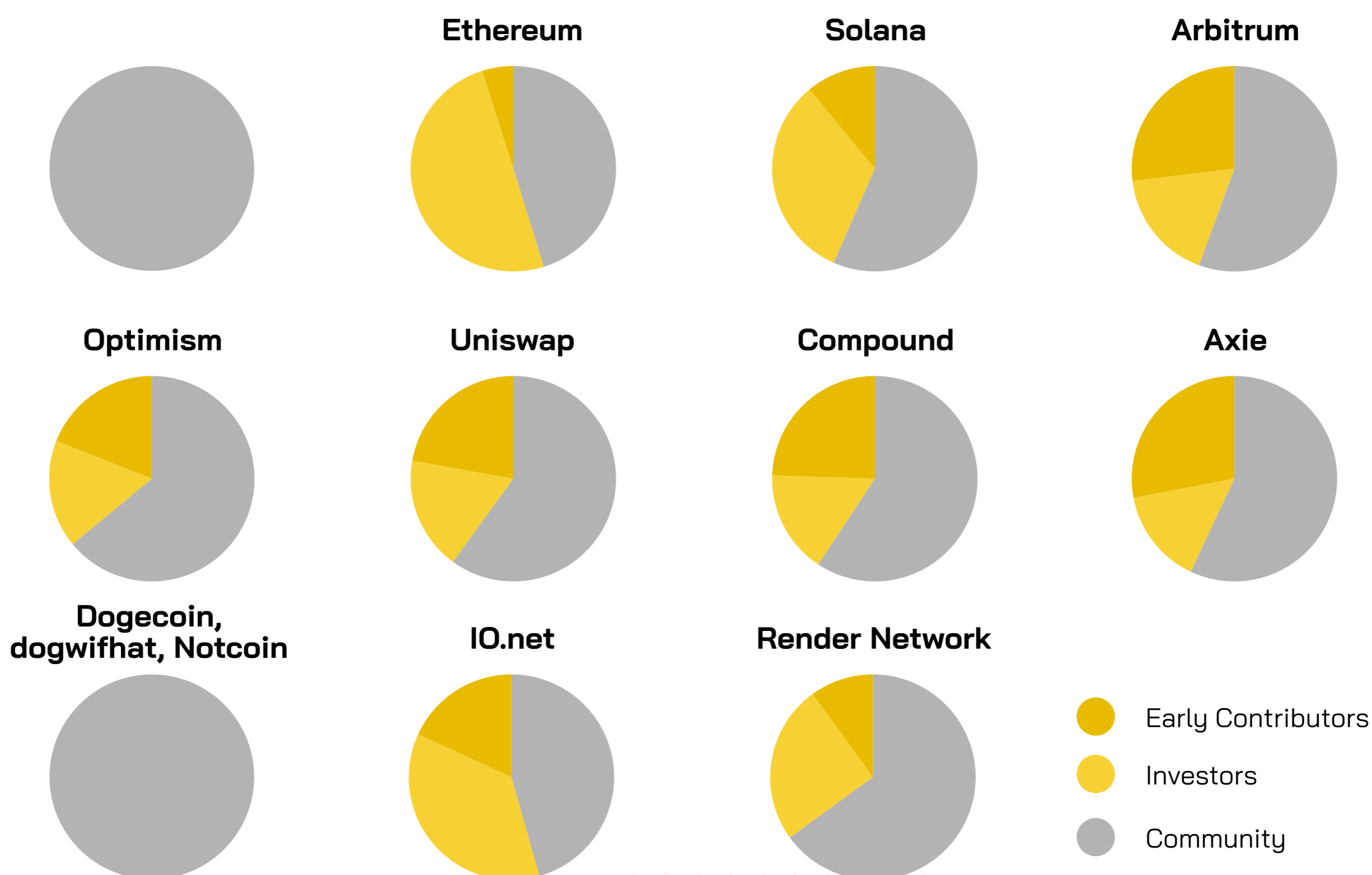
Hình 6: Tỷ lệ phân bổ token của một số dự án nổi bật
