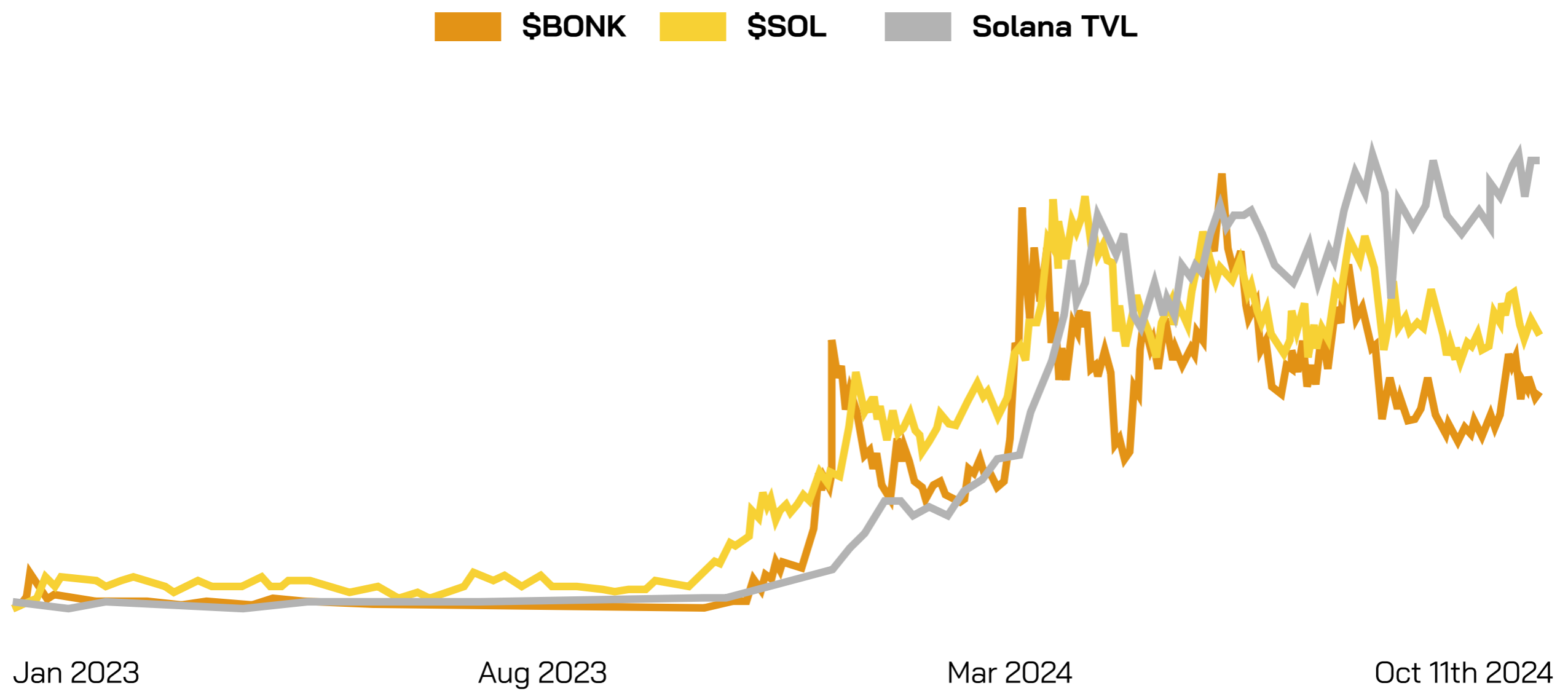
Hình 7: Sự tương quan giữa giá BONK, SOL và TVL của Solana
