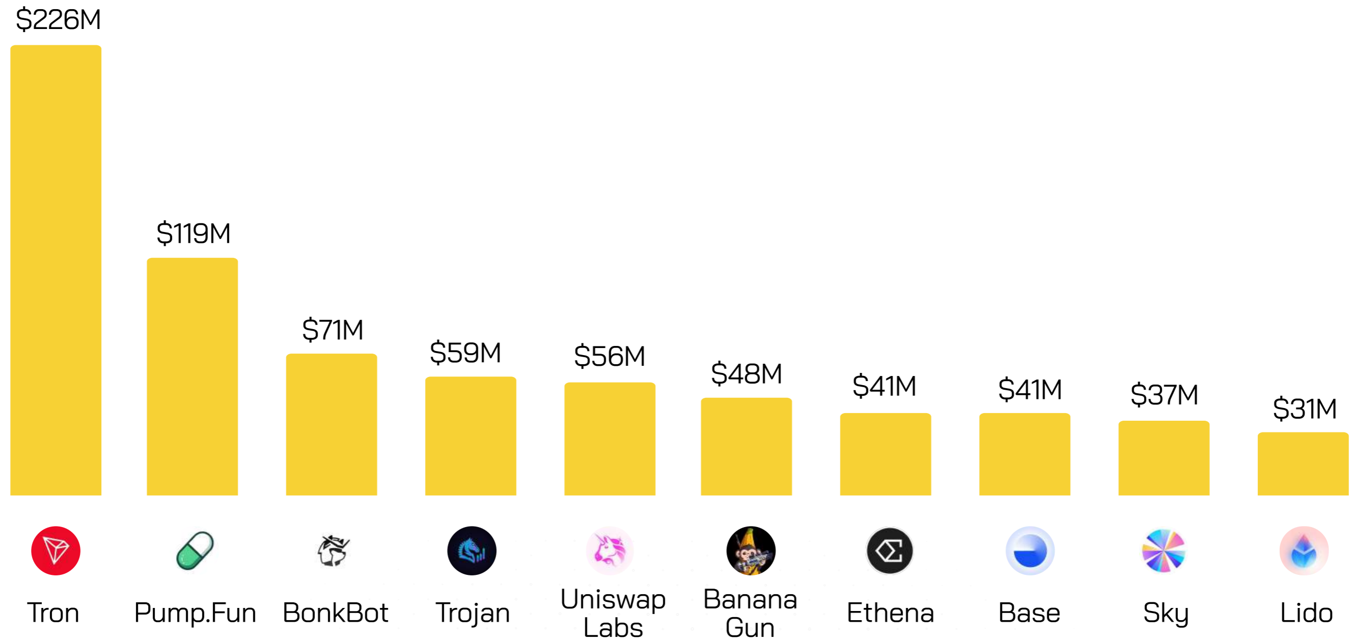
Hình 18: Top 10 dự án có lợi nhuận tích lũy cao nhất từ đầu năm 2024 đến nay
