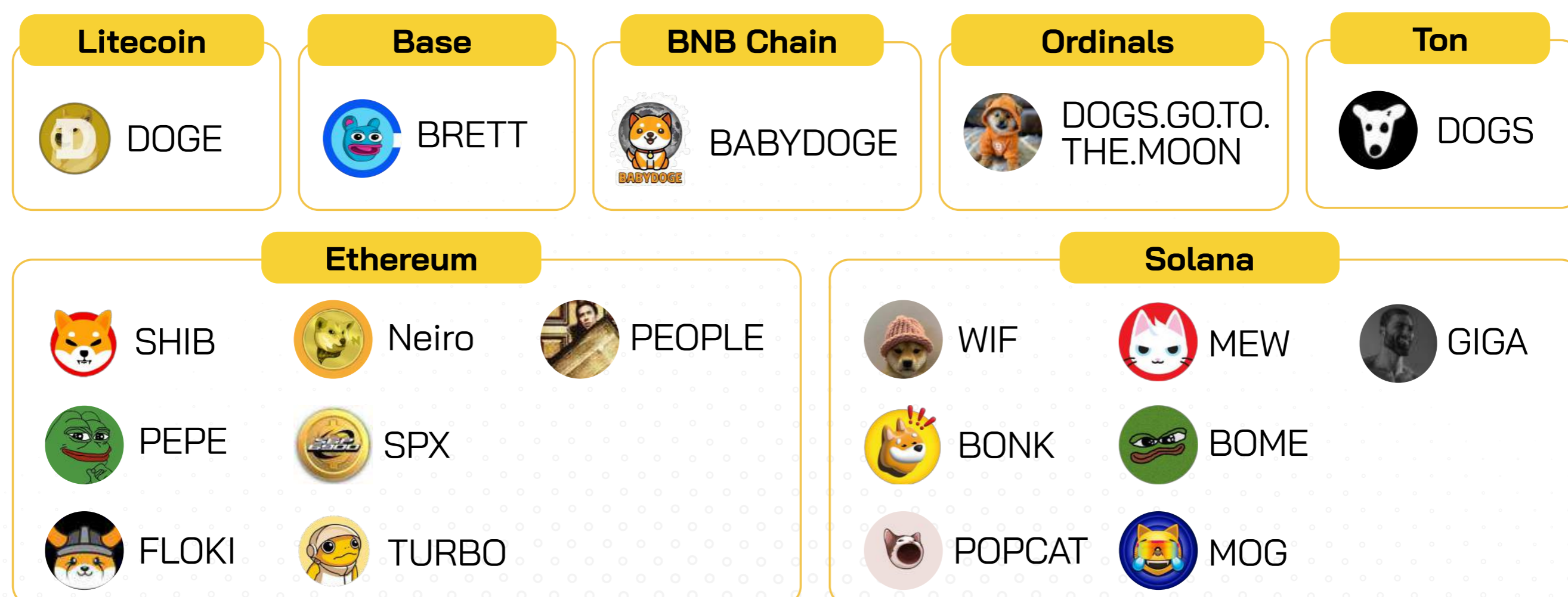
Hình 14: Meme coin có vốn hoá lớn nhất trên một số hệ sinh thái phát triển
