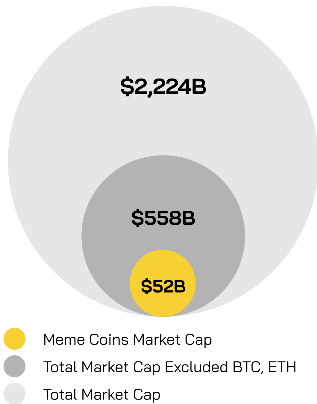
Hình 11: Bảng thông số thị trường meme coin và 10 meme coin hàng đầu
